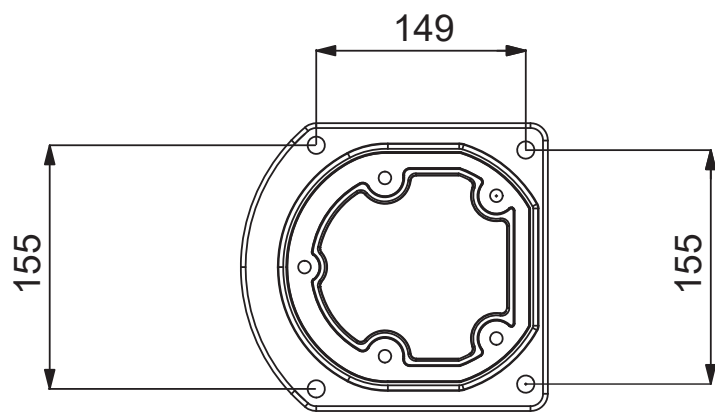
Sezione scala / section, scale 1:5
